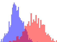
Klassifikation
