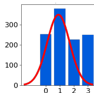
Statistik
