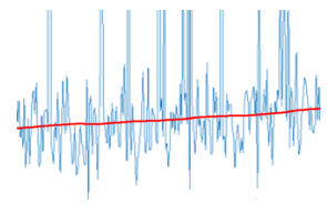
Zeitreihenanalyse
