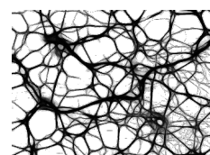
Neuronale Netze
