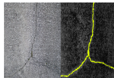
Bildanalyse
